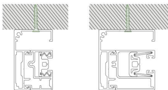
1. guide fissate frontalmente
